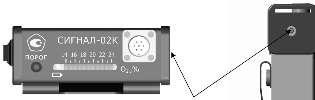
Рис.2. Место пломбирования.
