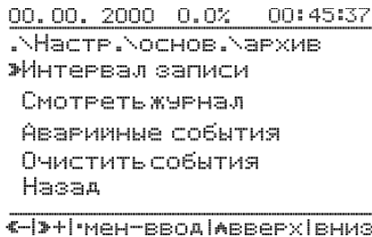
Рисунок 2.16 – Окно «Архивирование»
